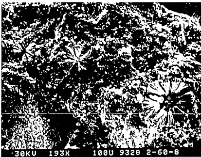
Fig. 4.- Gel de ASR y ettringitas
