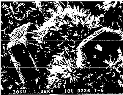
Fig. 3.- Portlanditas
